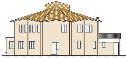
PROSPETTO NORD
