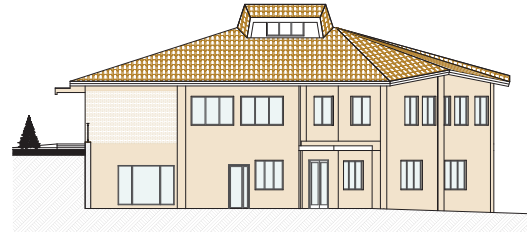
PROSPETTO OVEST
